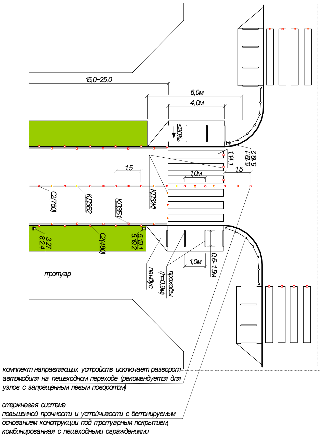
Рисунок 14 – Ограничение доступа автомобилей к пешеходным переходам в зоне перекрестка
